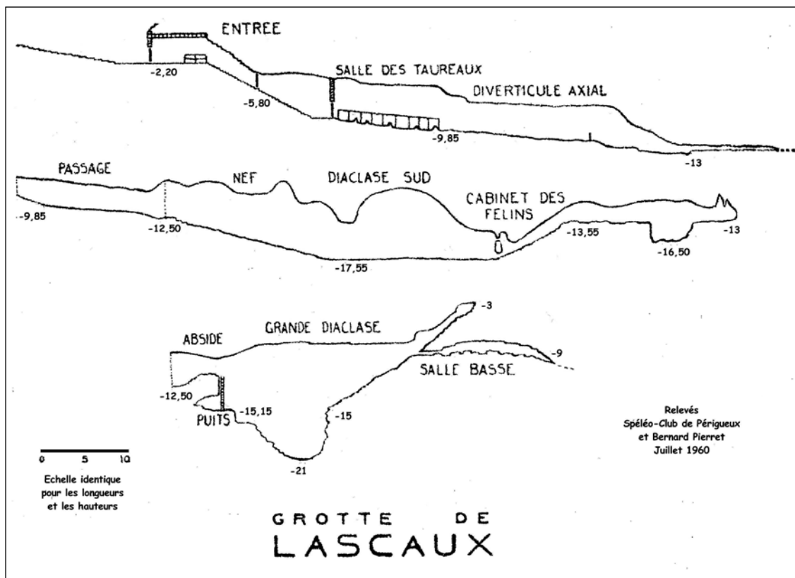
Fig. 2. Grotte de Lascaux. Coupe longitudinale Entrée - fond du Diverticule axial ; coupe longitudinale Passage - Nef - Galerie des Félines ; coupe longitudinale Abside - Puits - Salles ensablées, nommées ici Salle Basse. Relevés Spéléo-Club de Périgueux et Bernard Pierret. Mise au propre par Bernard Pierret. Juillet 1960.
