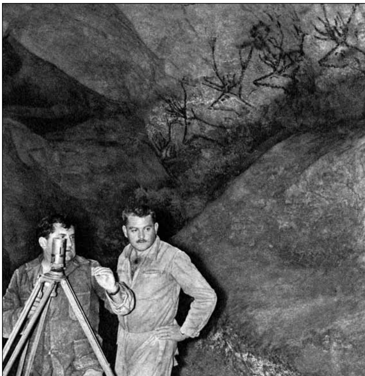
Fig. 1. Robert de Faccio et Bernard Pierret lèvent le plan et les coupes de Lascaux au théodolite en 1960 (photo J. Lagrange).
